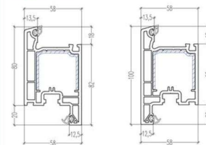
Hoja Apertura Interior 100mm 103.066 Refuerzo 113.147 Hoja Apertura Exterior 100mm 103.219 Refuerzo 113.147
