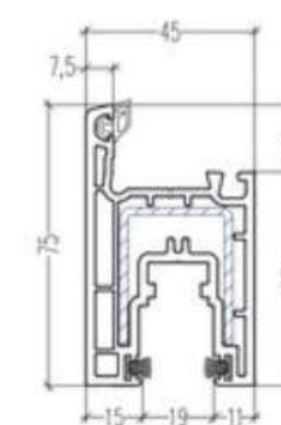
Hoja Corredera 75mm 105.322 Refuerzo 113.034
