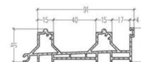
Solera Aluminio 31mm 104.328
