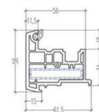
Batiente 58mm 102.196 Refuerzo 113.013
