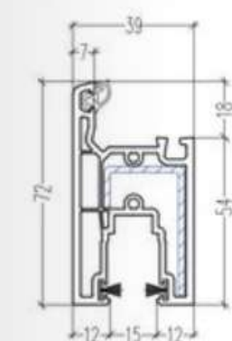
Hoja Corredera 72mm 105.378 Refuerzo 113.444.3
