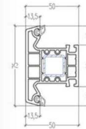
Travesaño 75mm 102.321 Refuerzo 113.032
