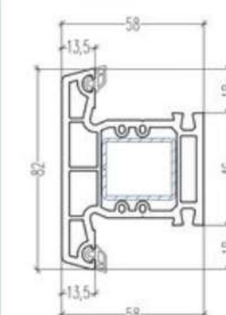
Travesaño 82mm 102.113 Refuerzo 113.002
