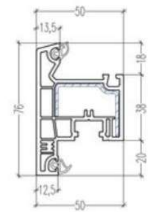
Hoja Apertura Exterior 76mm 103.361 Refuerzo 113.384
