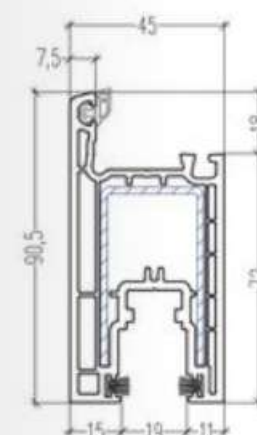
Hoja Corredera 90,5mm 105.135 Refuerzo 113.043
