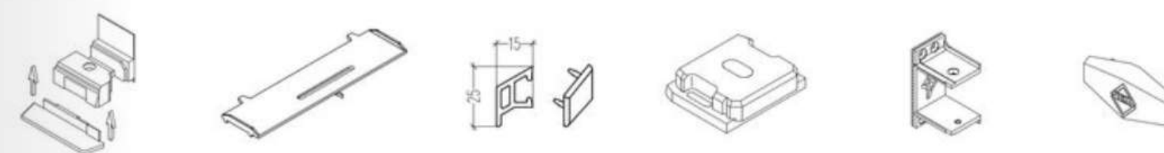
Remate Batiente 109.584 Puente Acristalar 109.293 Vierteagua 109.030 Tapa 109.140 Zapata Estanquidad 106.013 Escuadra Unión Travesaño 106.016 Tapa Desagüe 109.053
