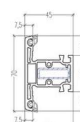
Travesaño 70mm 105.326 Refuerzo 113.020
