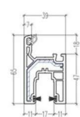
Hoja Corredera 65mm 105.373 Refuerzo 113.074
